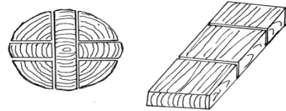
Şekil 1. Deney Örneği Kesim Planı
